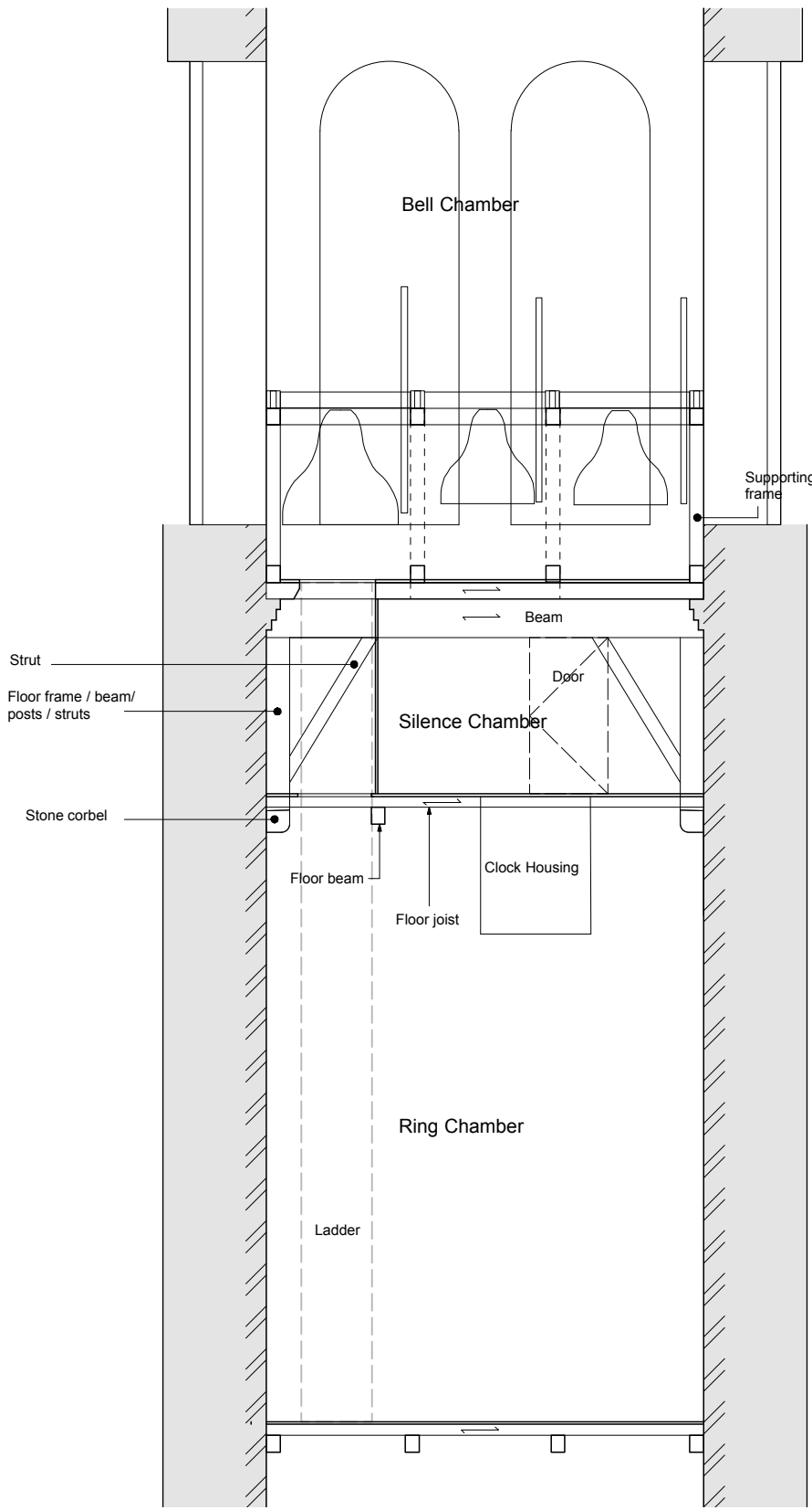
SECTION A-A
